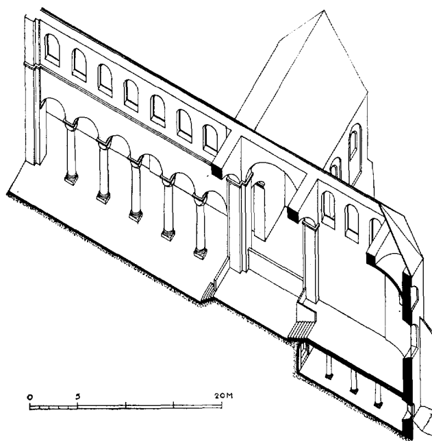
Fig. 2. Utrecht, St. Pieter. Reconstructie oorspronkelijke toestand. (Bij gebrek aan voldoende gegevens is de westerpartij niet getekend.) (Tek. H. W. van der Voet.)
